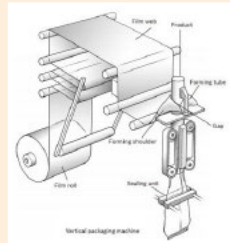
Schlauchbeutelmaschine
